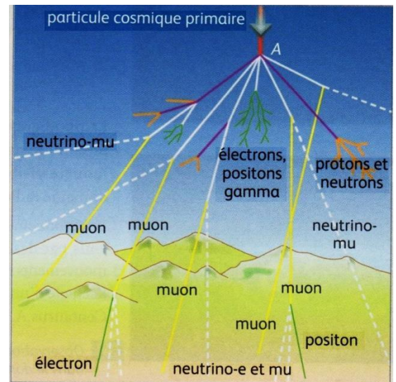
Gerbes de particules issues du rayonnement cosmique
